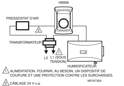
Fig. 15. Raccordement du H8908 en série avec pressostat d'air et humidificateur.
