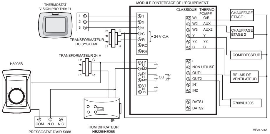
Fig. 17. Raccordement du H8908 avec un VisionPRO® IAQ sur un système de chauffage typique à deux étages.
